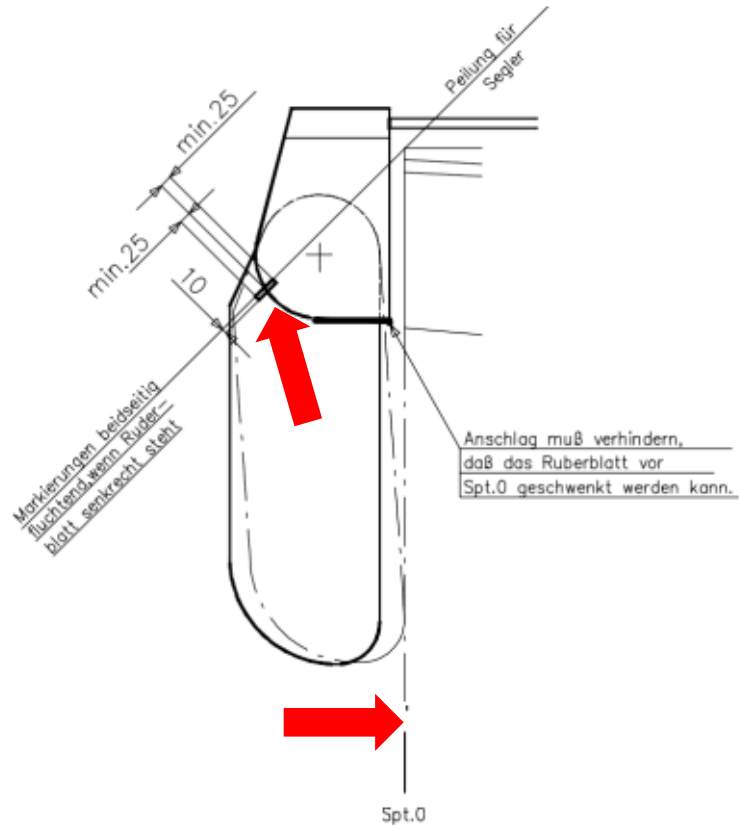
Abb. 13: Absenkung Ruderblatt
