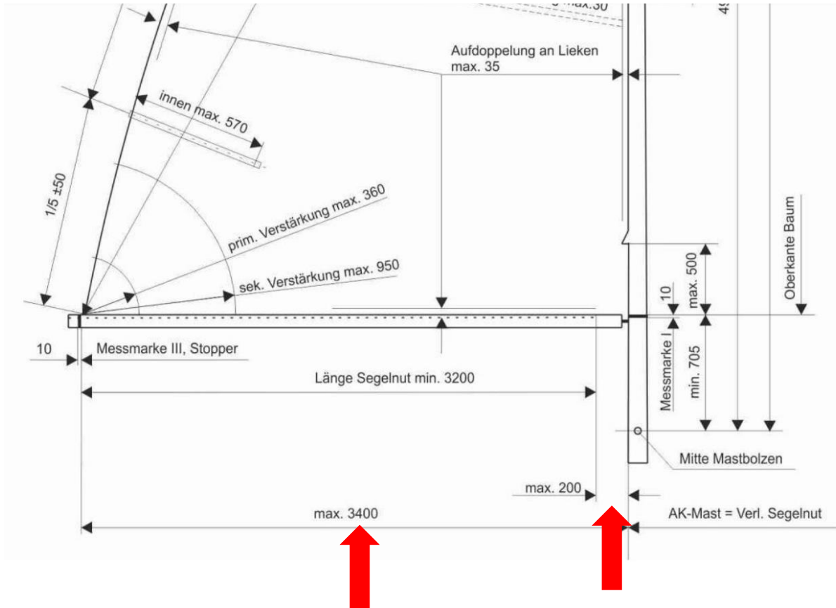
Abb. 15: Mast, Großbaum, Stehendes und Laufendes Gut, Segel
